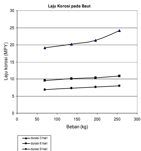
Grafik 8. Pengaruh Tegangan Dalam Terhadap Laju pada Baut
