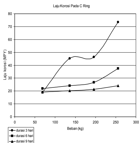
Gambar 7. Pengaruh Tegangan Dalam Terhadap Laju Korosi pada C ring
