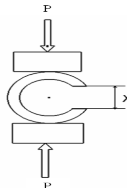
Gambar 4. Metode pembebanan pada benda uji bentuk C-ring
